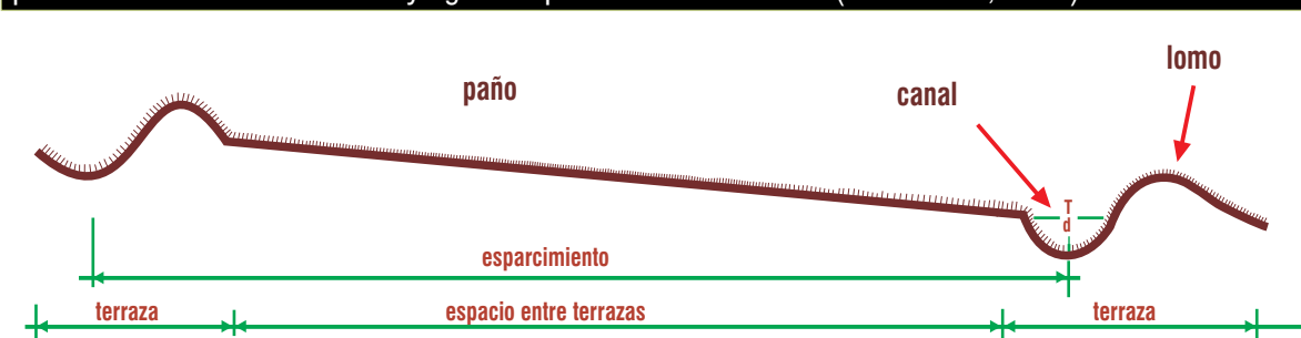
Figura 4. Terraza y sus componentes. Modificado de Manual de sistematización de tierras para control de erosión hídrica y aguas superficiales excedentes (Scotta et al , 1989).
