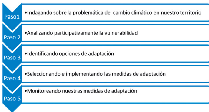
Esquema 4: cinco pasos para adaptarnos al cambio climático en nuestros territorios
