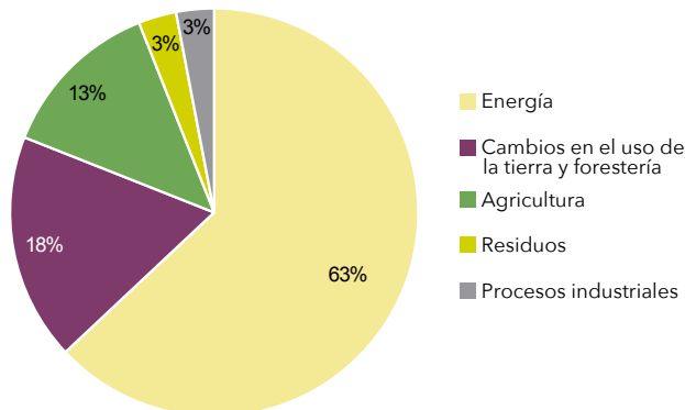
Gráfico 2: Proporciones de los diferentes sectores en la producción global de gases invernadero antropogénicos en el año 2000
