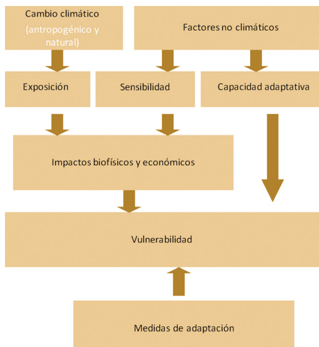
Esquema 1: Concepto de vulnerabilidad
