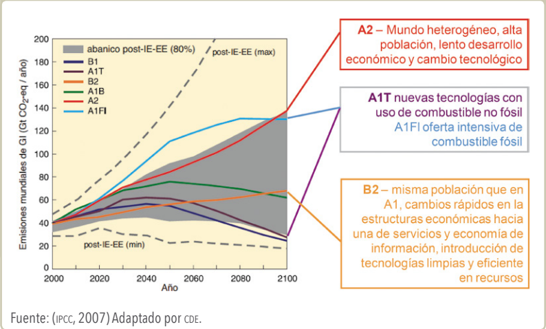
Gráfico 3: Tratando de mirar al futuro. Escenario de emisiones
