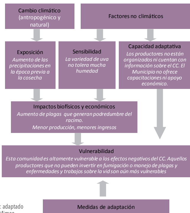
Esquema 2: vulnerabilidad en una plantación de vid
