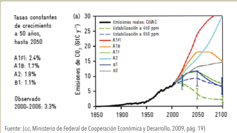
Gráfico 1: Emisiones de carbono (1850-2100)
